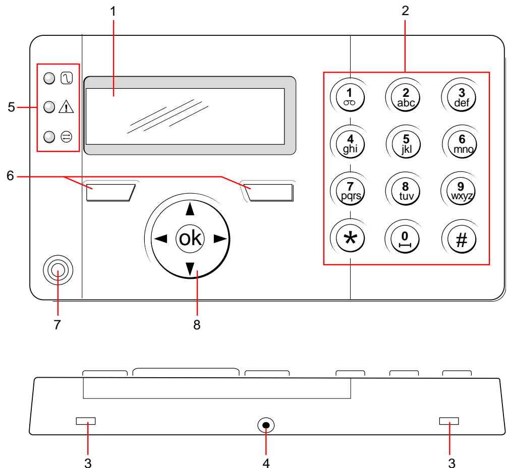
LCD-Bedienteil
