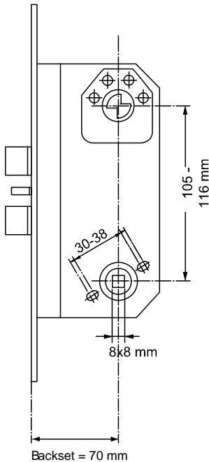
Fig. 3 CD30 door mounting
